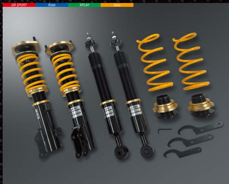
フロント キャンバー角調整式 ピロアッパーマウント
